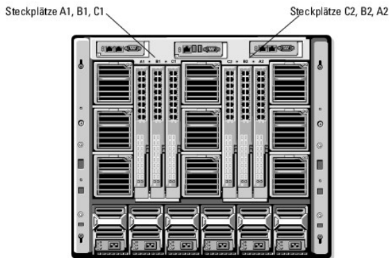
Abbildung 10-1. Rückansicht eines Gehäuses mit ausgewiesenen E/A-Modulpositionen
